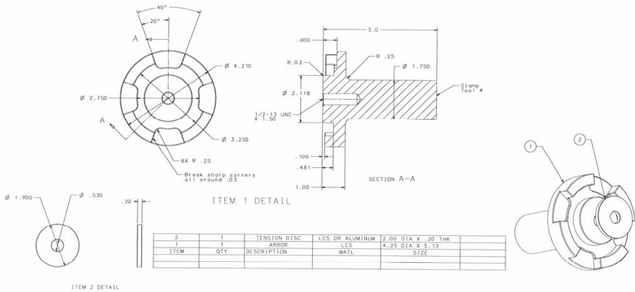
CFR / ETFE Impeller Trim Arbor (PT0827) Fig. 11-9
