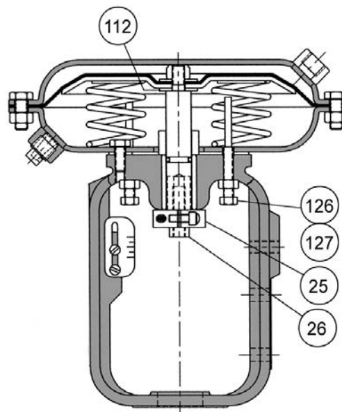
Figura 9. Actuador Baumann 32 con tope dual, extensión neumática (ATE)
