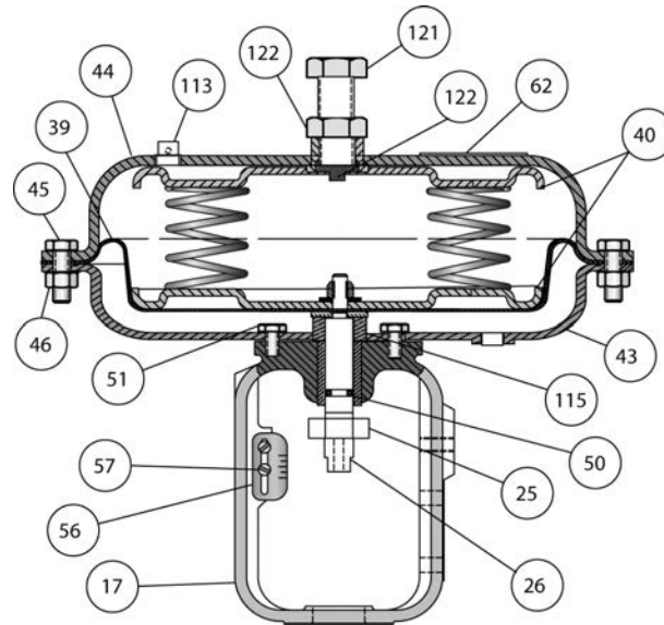
Figura 14. Actuador Baumann 70
