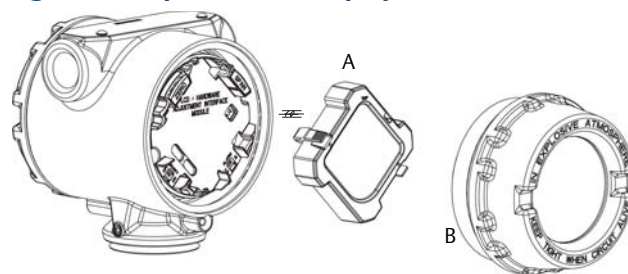
A. LCD display B. Meter cover
